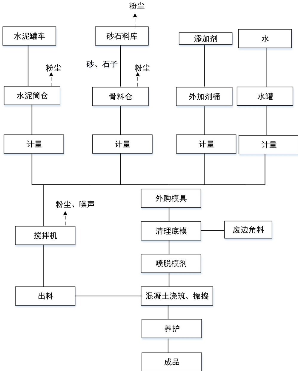
图 5 砼四脚体预制构件生产线工艺流程及产污环节简图
