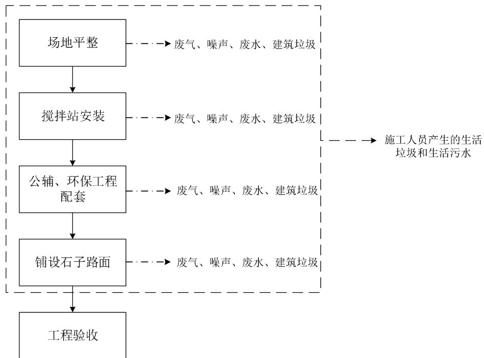
图 2-3 工艺流程及产污环节示意图
