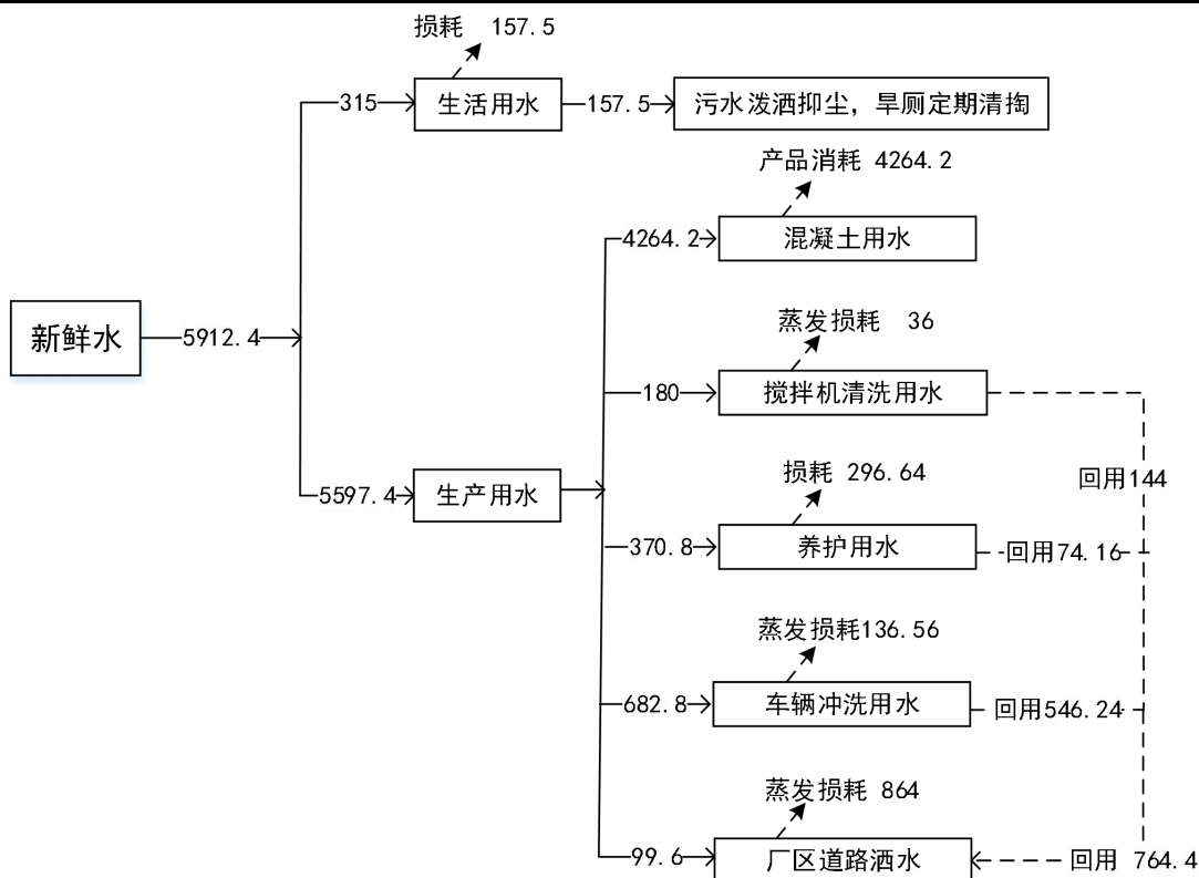
图 2-1 水平衡关系图 (单位: m³/a)
