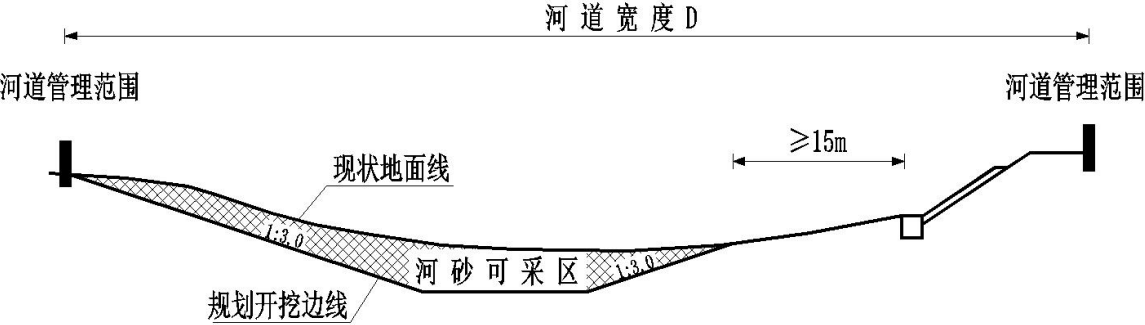
图 6.3-2 单侧护岸河道可采区划定示意图
